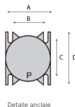
Detalle anclaje
