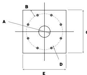
Detalle anclaje
